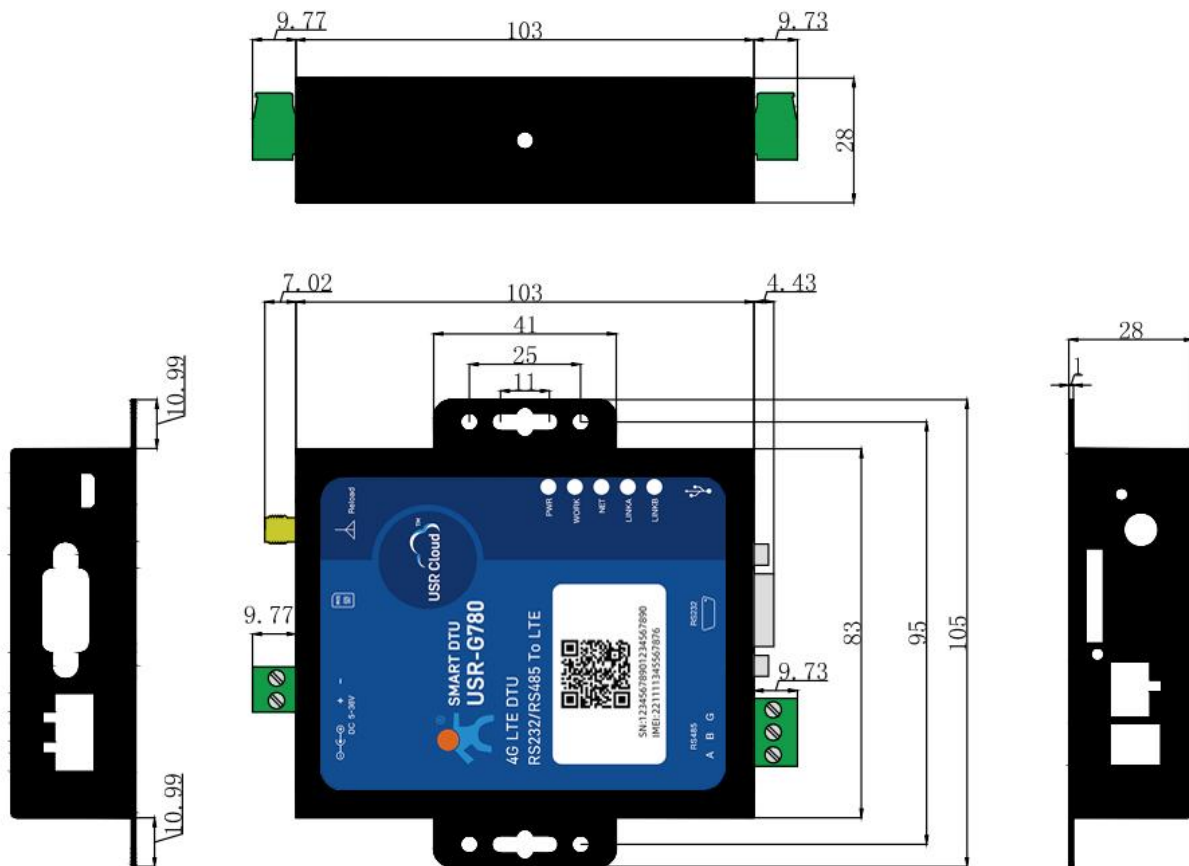
图 1. USR-G780 尺寸图
